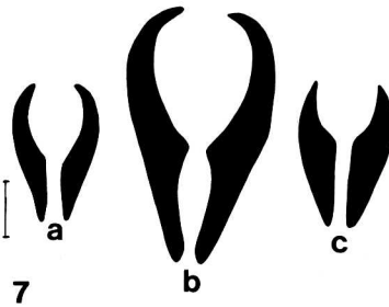
Abb. 6. Doppelhaken von Acanthoteuthis leichi n. sp. Maßstab 1 mm (gilt für Abb. 6–9). a) Distal, b) zentral, c) proximal.
