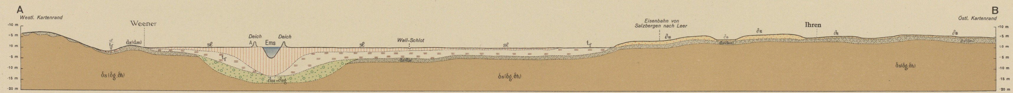
Schnitt A-B vom Westrand über die Ems zum Ostrand des Blattes Längen 1:25000, Höhen 1:1000
