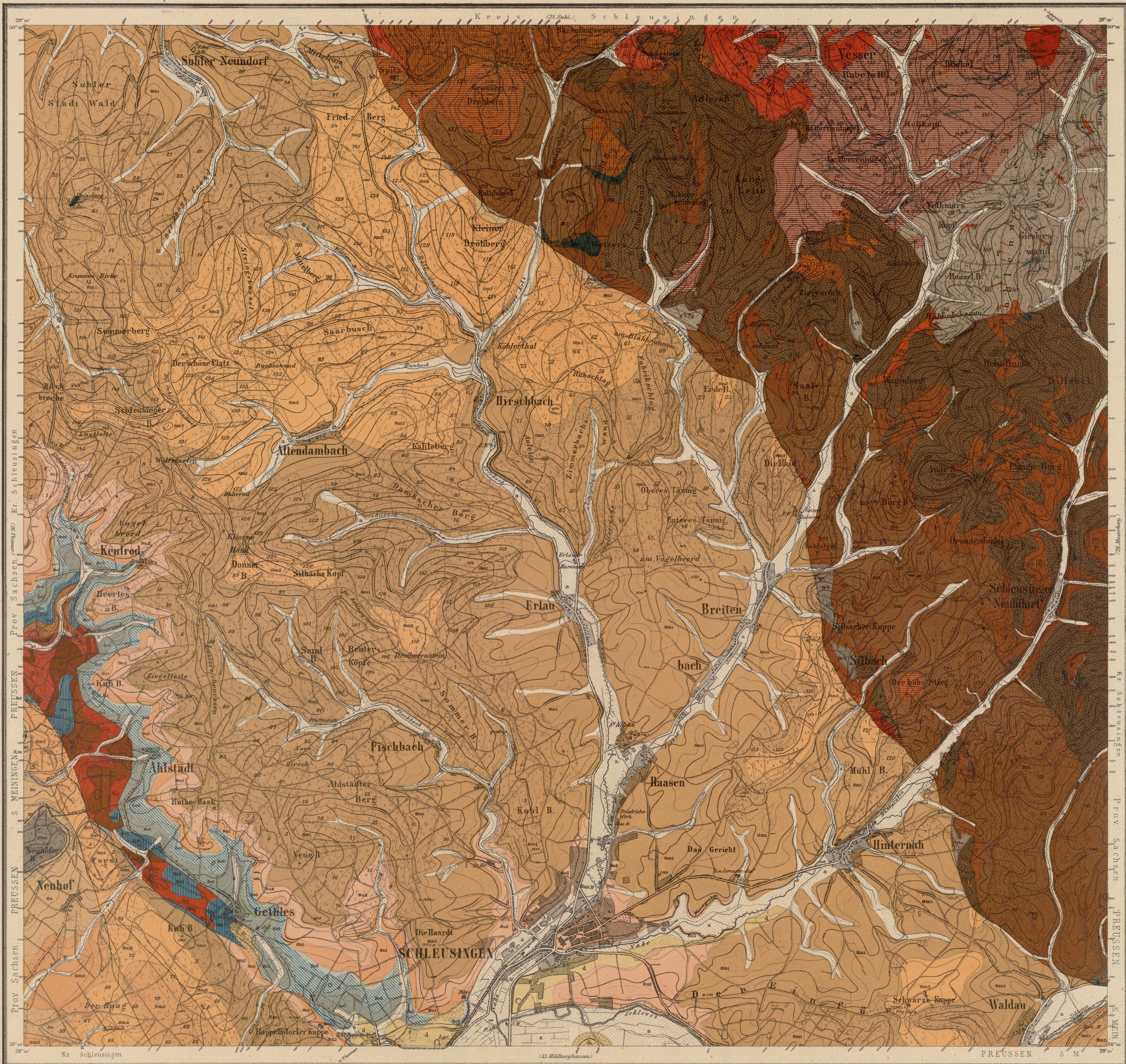
Topogr. Aufnahme des kgl. Preuss. Generalstabes 1856. Nachträge bei der geologischen Aufnahme. Herausgegeben von der kgl. Preuss. geol. Landesanstalt 1898. Lieferung 67.
