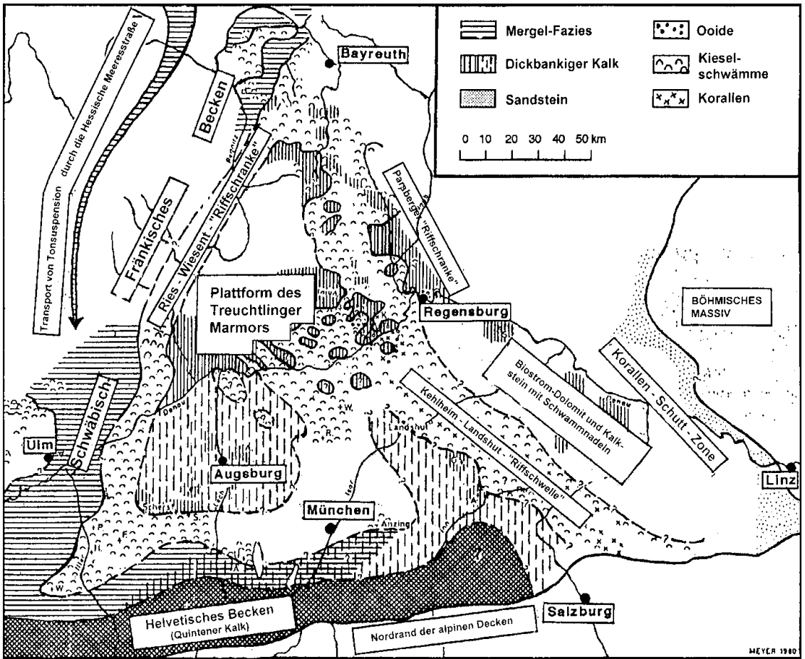
Abb. 4: Die Karbonatplattform des Treuchtlinger Kalksteins (»Marmor«) nach MEYER & SCHMIDT-KALER (1990a).
