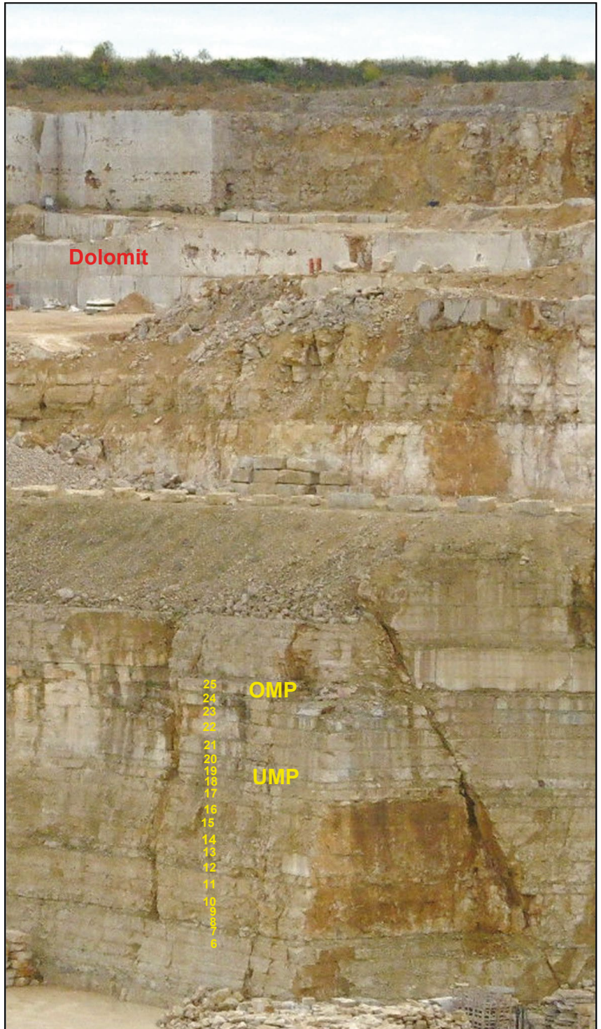
Abb. 3: Die Bankfolge des Treuchtlinger Kalksteins im Steinbruch Frankenschotter bei Treuchtlingen mit Nummerierung der Schichten gemäß BEYER & GRIMM (1997). Die Untere (UMP) und Obere Mergelplatte (OMP) sind markiert. Das obere Drittel der etwa 60 m mächtigen Abfolge besteht in diesem Steinbruch aus Dolomit (dolomitisierte Dickbank-Kalke).
