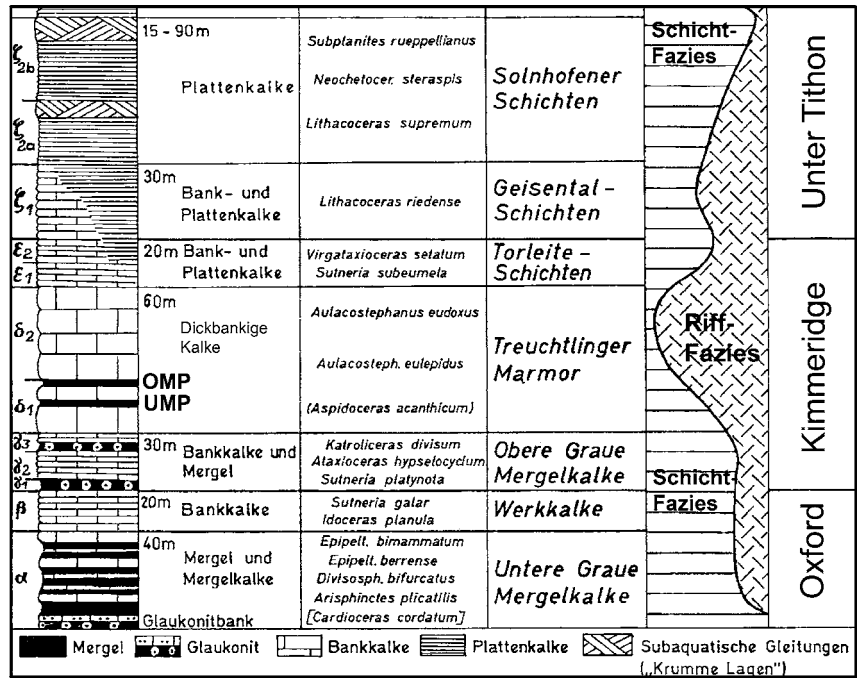
Abb. 5: Ausschnitt des Bereichs der Unteren und Oberen Mergelplatte aus dem Schema der Malm-Stratigraphie in der Südlichen Frankenalb (aus ZEISS 1977).
