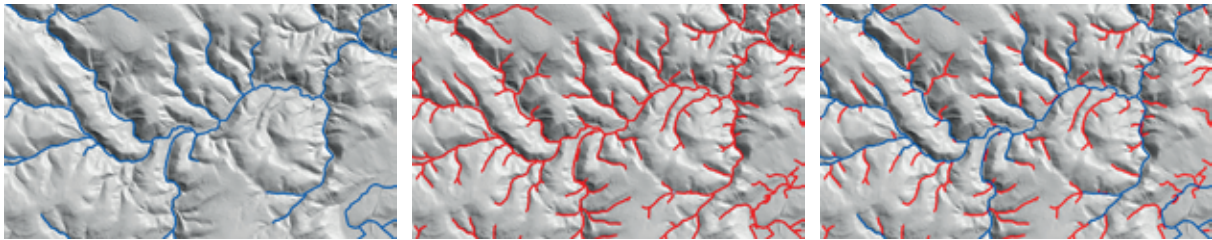
Abb. 5: LfU-Gewässernetz 9841 (links), Tiefenlinien (Mitte) und erweitertes Gewässernetz (rechts).
