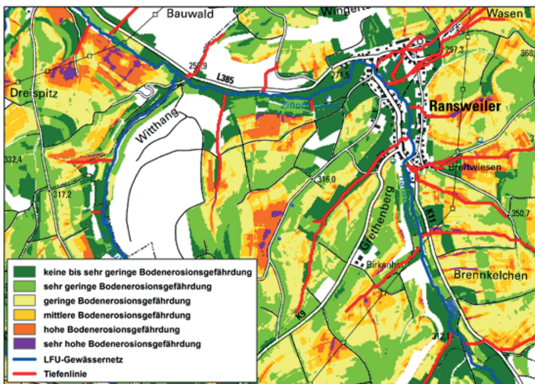
Abb. 9: Anschluss erosionsgefährdeter Flächen an das erweiterte Gewässernetz.
