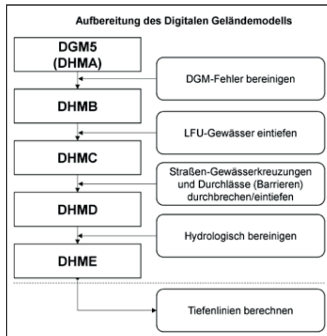
Abb. 4: Schema der Aufbereitung des DGM5.
