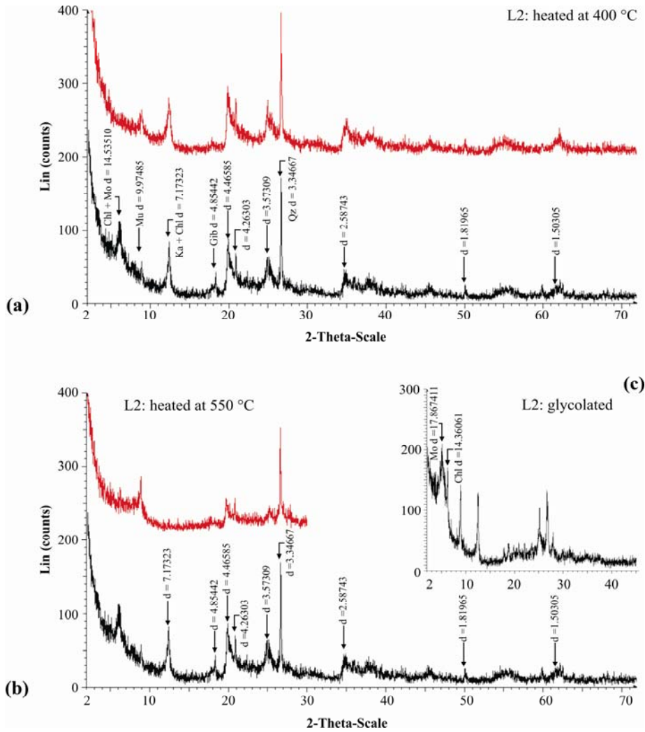
Abb. 23. Röntgendiffraktogramme der Sektion Lava. (a) Probe 2 bei 400 °C, (b) bei 550 °C getempert, (c) glykolisiert. Mu = Muskovit, Ka = Kaolinit, Mo = Montmorillonit, Qz = Quarz, Fd = Feldspat, Chl = Chlorite, Gib = Gibbsit.
