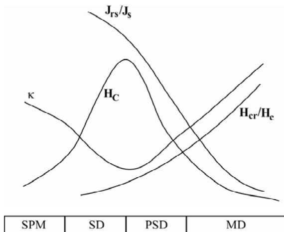
Abb. 16. Schematische Darstellung der Koerzitivkraft ( H_c ), der Suszeptibilität ( k ), der Sättigungsremanenz/Sättigungsmagnetisierung ( J_{rs}/J_s ) und der Remanenzkoerzitivkraft/Koerzitivkraft ( H_{cr}/H_c ) in Abhängigkeit von der Teilchengröße. Verändert nach Soffel (1991).
