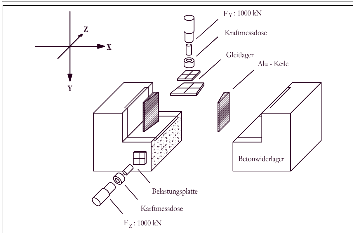
Abbildung 5-7: Gefügeversuchstand „Reiche Zeche“ in Schnittdarstellung
