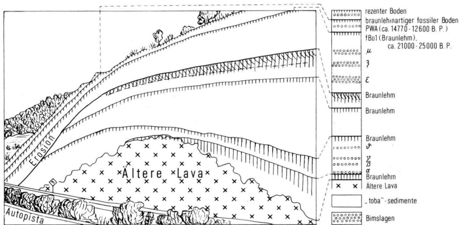
Abb. 4. Die Zeichnung zeigt den gleichen Profilausschnitt wie das Photo der Abb. 3. Das schematische Profil der Schichten (rechts) macht die enge Beziehung zwischen Bimsapilli-Lagen und „toba“-Sedimenten deutlich. Die Ablagerungen unter dem fossilen Boden fBo1 haben ein Alter über rund 25 000 Jahre vor heute. Auf dem Photo (Abb. 3) sind die Bimslagen nicht zu erkennen, da infolge von Abspülungsprozessen „toba“-Material die Aufschlußwand überzieht.
