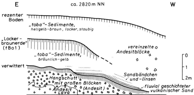
Abb. 7. Profil am Nordosthang der Iztaccíhuatl an der Straße (Libre) von Texmelucan zum Rio Frio-Paß. Über Andesitlava befindet sich Hangschutt, darauf — durch einen fossilen Boden gegliedert — „toba“-Sedimente. Vgl. die Erläuterungen im Text.
