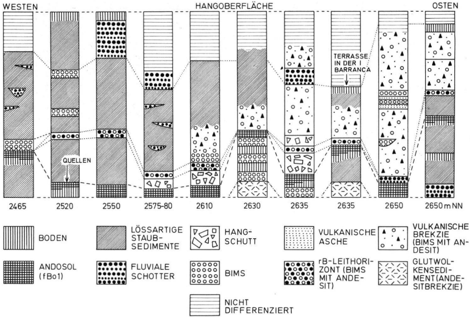
Abb. 2. Profile der Barranca Xotanacatla am Malinche-Westhang zwischen 2650 und 2465 m NN. Stratigraphisch wichtige Horizonte sind der fossile Boden fBoI und das Bimslapilli-Band mit Andesitfragmenten (rB).
