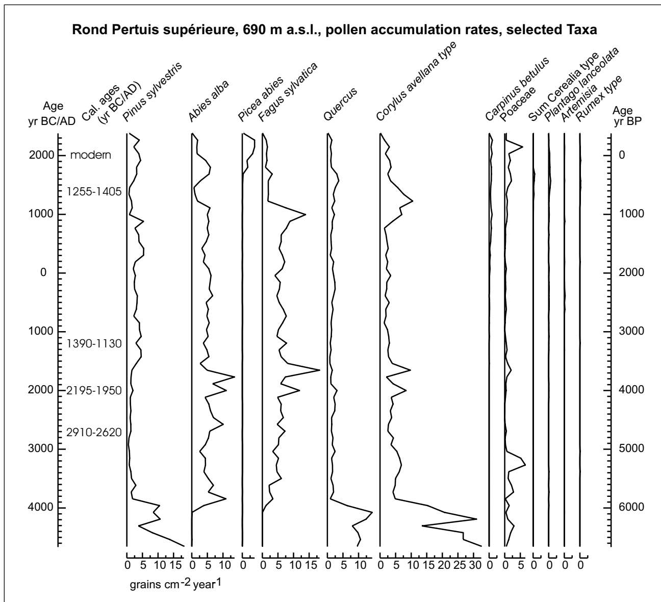
Fig. 4: Pollen accumulation rates from the Rond Pertuis supérieure bog, Northern Vosges, France, 690 m a.s.l. with selected Taxa. Abb. 4: Raten des Pollenniederschlags für ausgewählte Taxa des Rond Pertuis supérieure, Nordvogesen, Frankreich, 690 m ü. NN.
