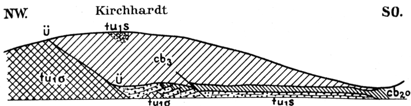
Schematisches Profil an der Kirchhardt im Salchbachtal.
