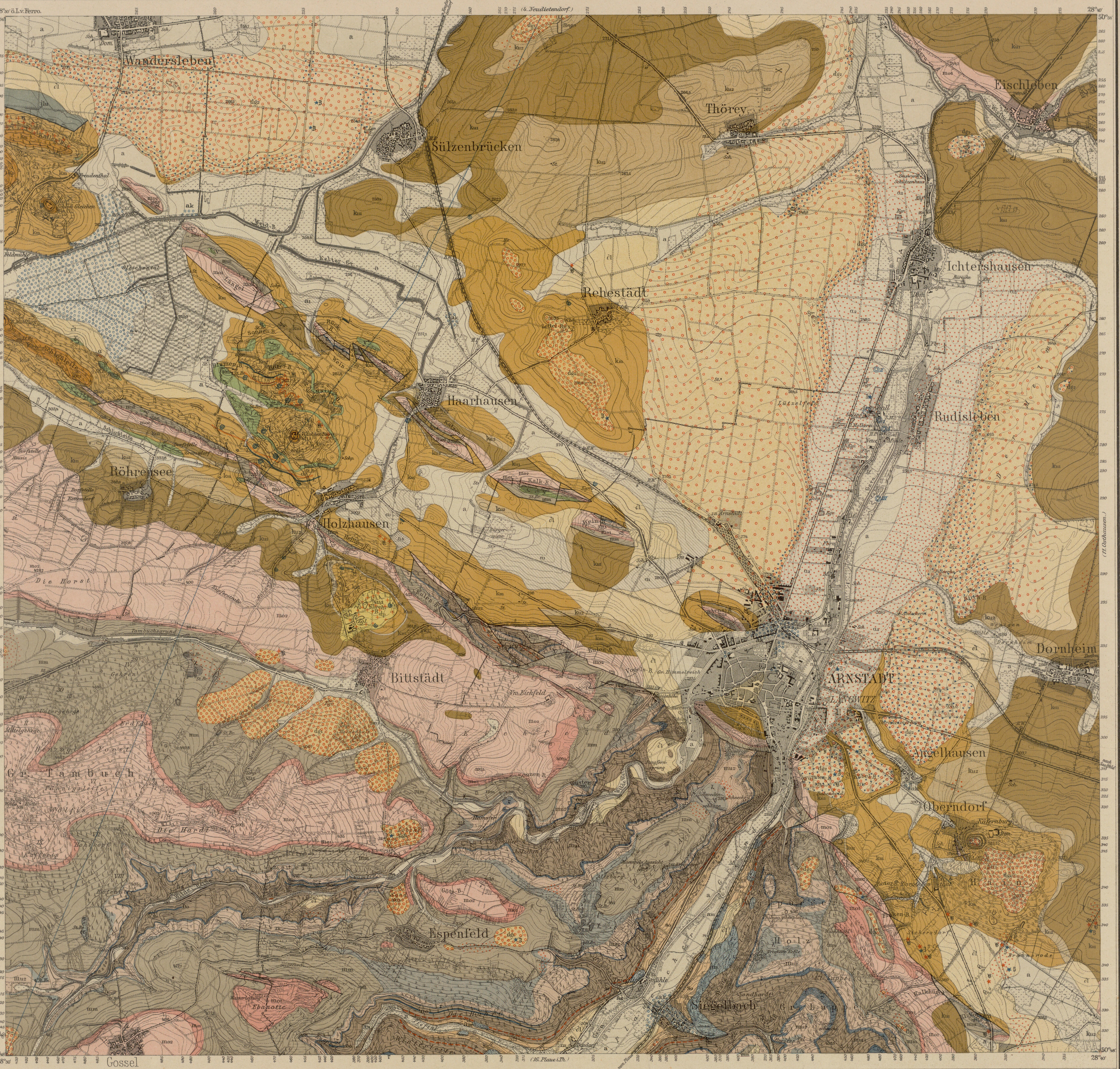
Topogr. Aufnahme des Preuß. Generalstabes 1903. Nachträge bei der geolog. Aufnahme. Herausgegeben von der Preuß. geolog. Landesanstalt 1920. Laufage geognostisch bearbeitet durch E.E. Schmid, 2. Auflage nach Begehungen von F. Zimmermann 1891 und 1919. Berliner Lithographisches Institut, Berlin W. 35.
