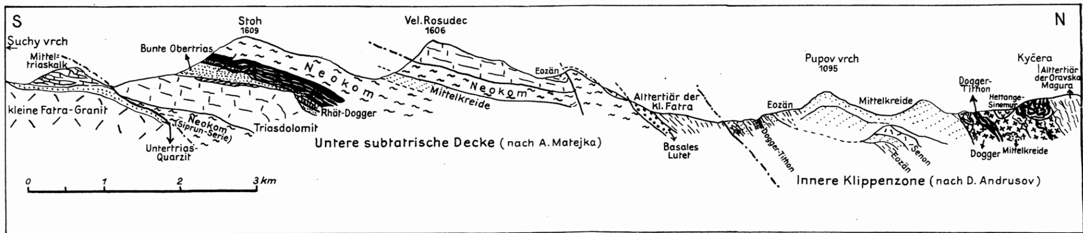
Abb. 87. Kräftige Südvergenz (spät- und nach-alttertiär) in den nordwestl. Zentralkarpaten. Nach Karpatenführer 1931. Atlas 2.
