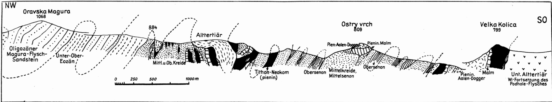
Abb. 85. Profil N. Dlha an der Orava der während bzw. nach dem Alttertiär gegen S bewegten Inneren Klippenzone. Nach D. ANDRUSOV 1931, Taf. XVII.
