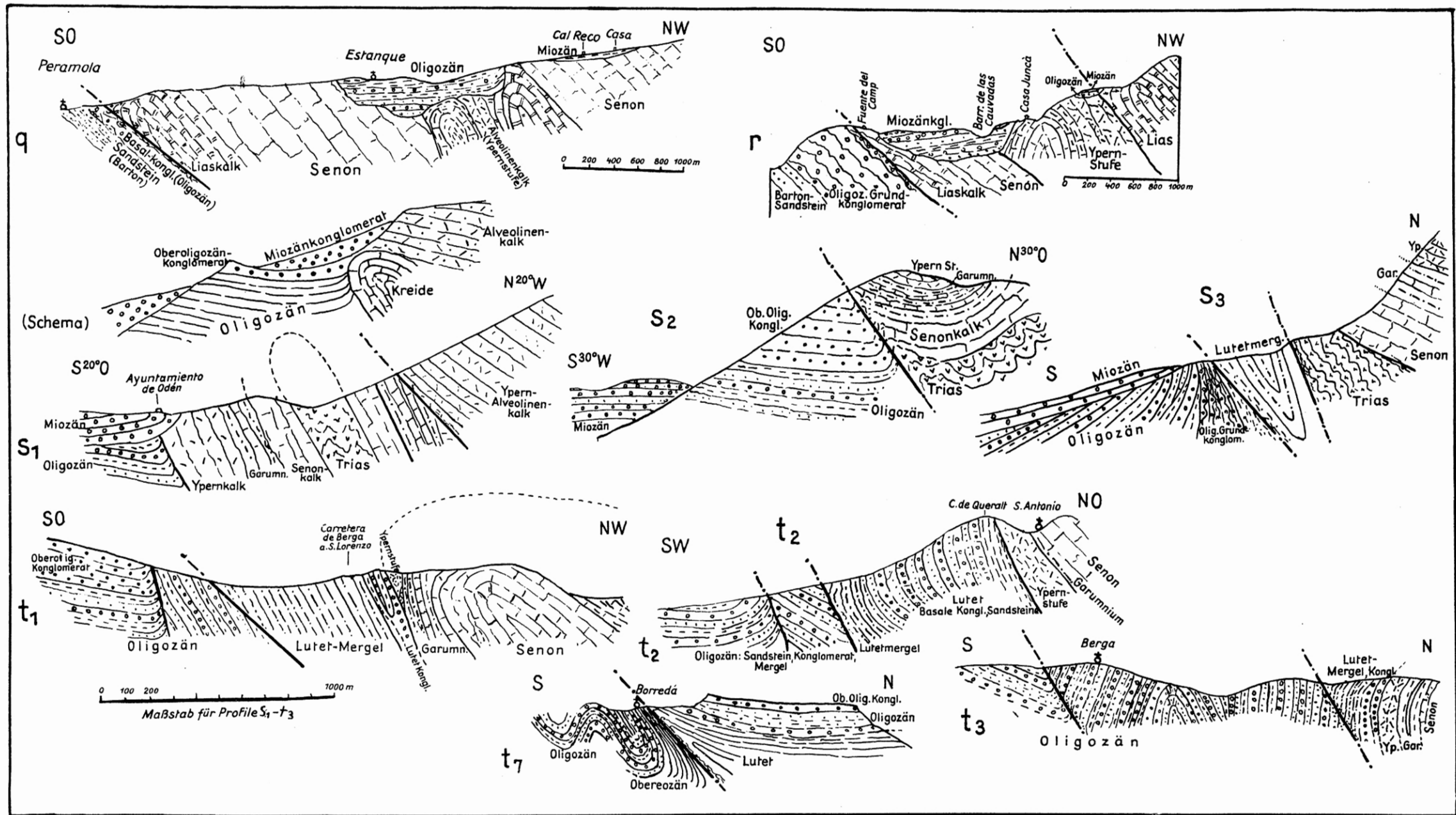
Abb. 59. Die Molasse am Pyrenäen-Südrand und ihr Bau. Umgezeichnet nach RIOS & ALMELA & GARRIDO 1943. Lage der Profile siehe Abb. 41, q—t.
