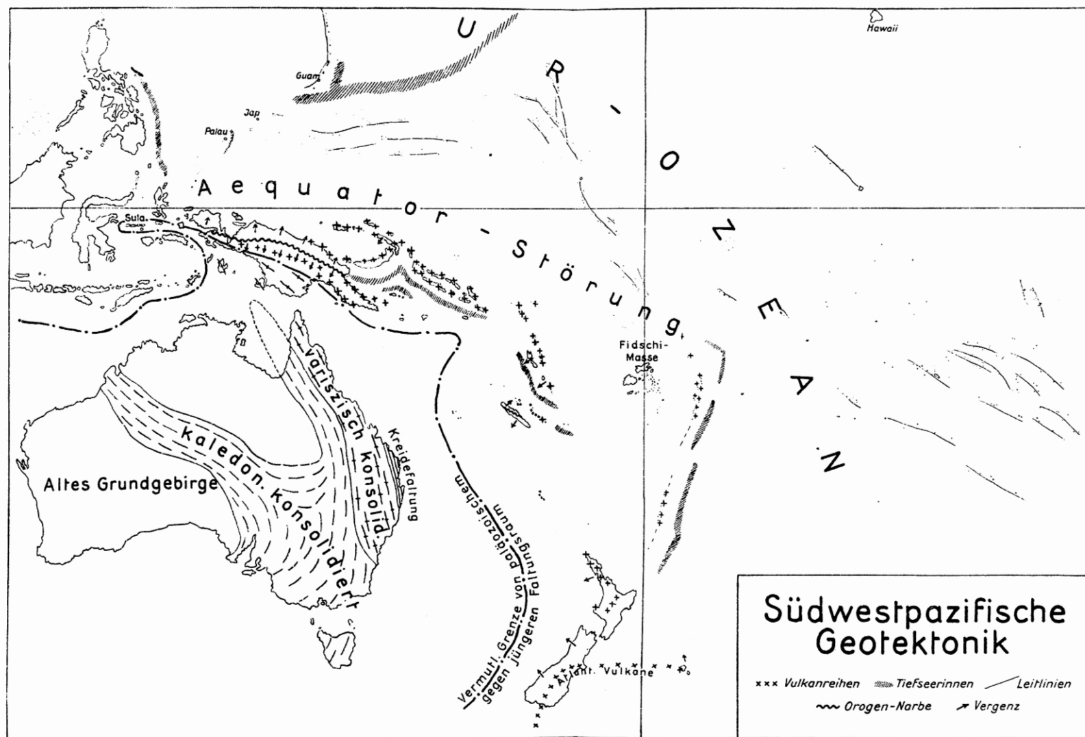
Abb. 130. Südwestpazifische Geotektonik. Kreuze: Vulkanreihen; schraffiert: Tiefseerinnen; einfache Linien: Leitlinien; Schlangelinie: Orogen-Narbe; Pfeile: Vergenzen.
