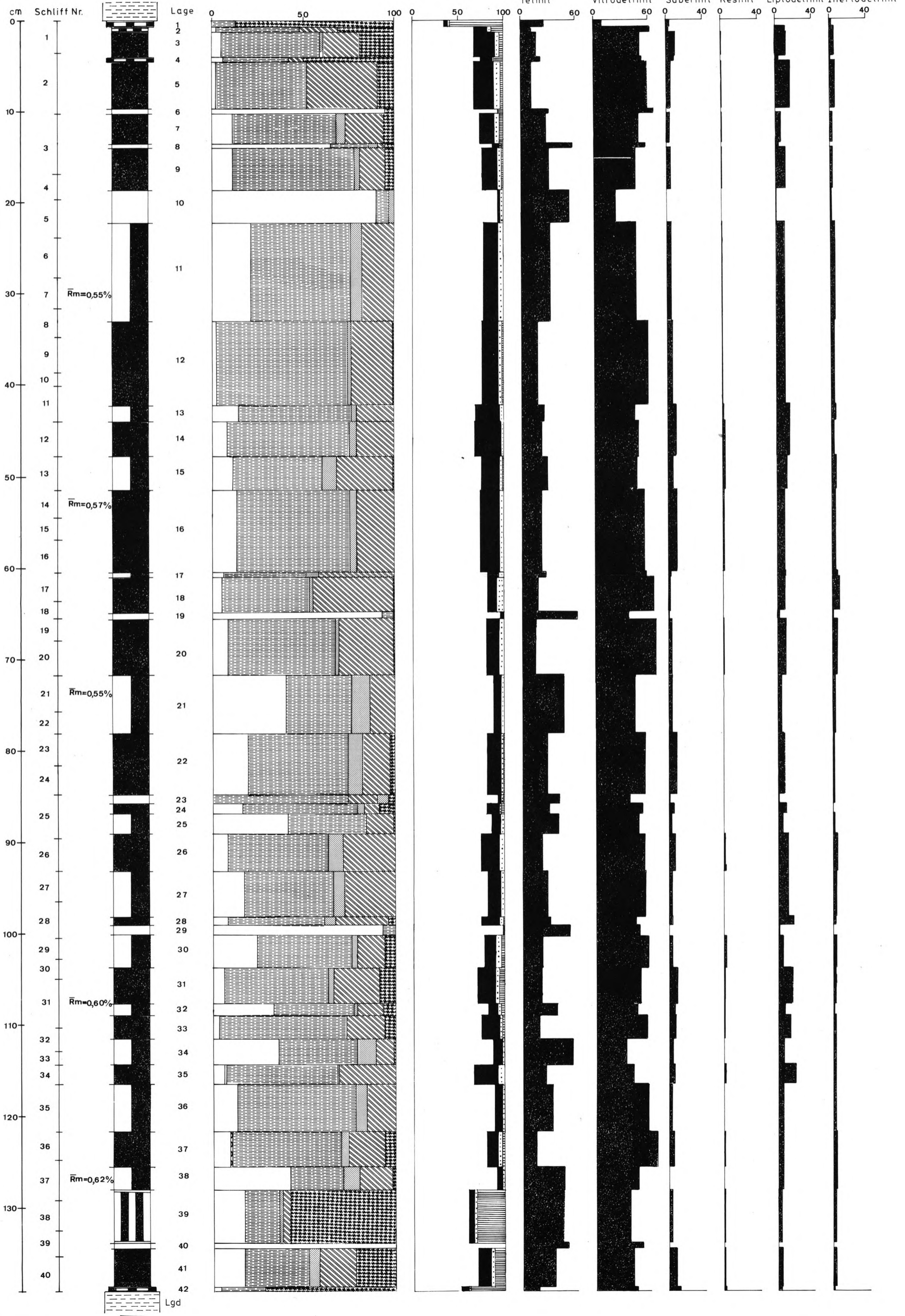
Analyse nach Mikrolithotypen (Vol-%)
