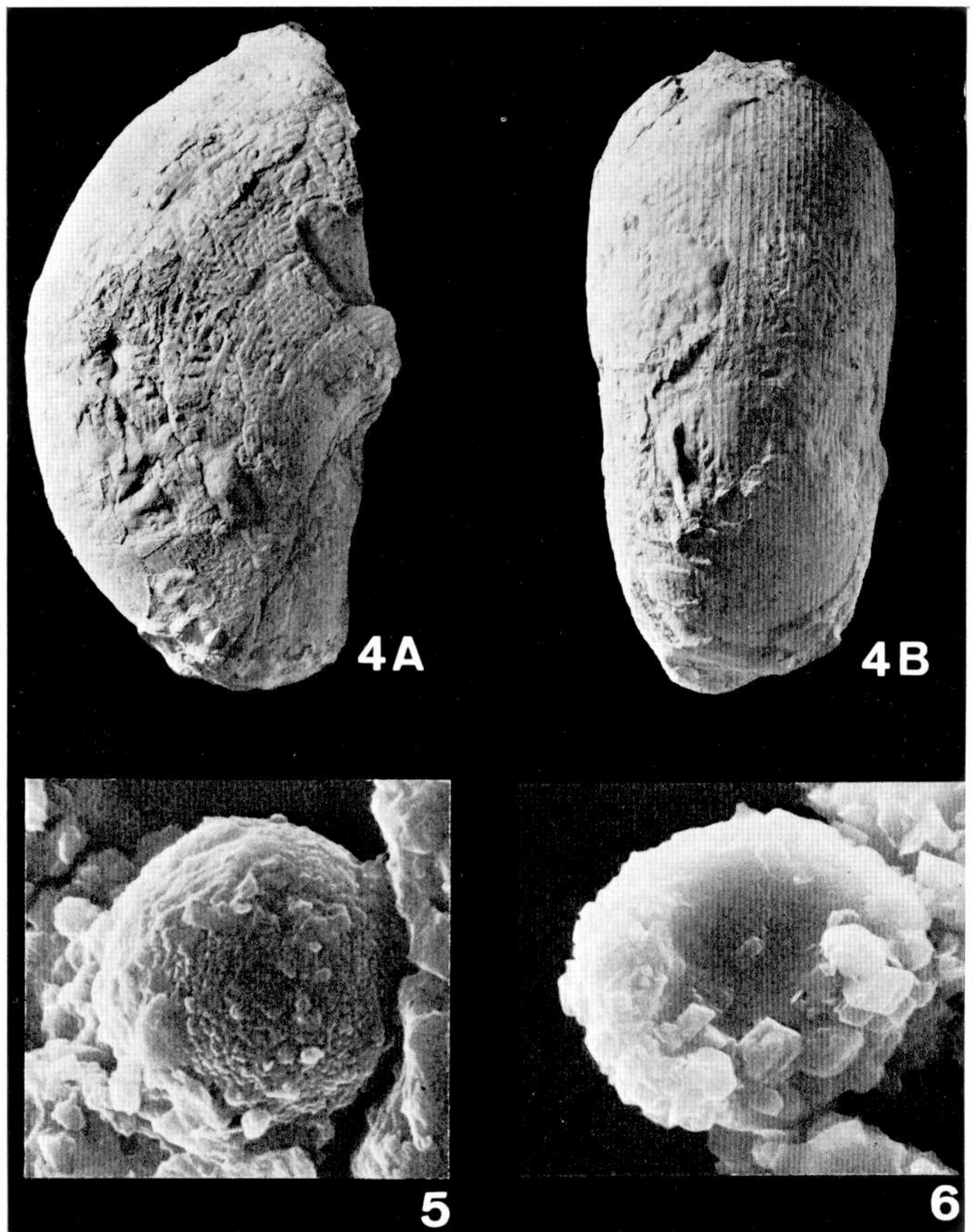
Abb. 4. Cladiscites cf. tornatus (BRONN). Exemplar GPIT 1546/2, Schicht La 97/76, Fundort wie 2. A. Lateral-, B. Ventralansicht, ca. 1/3.
