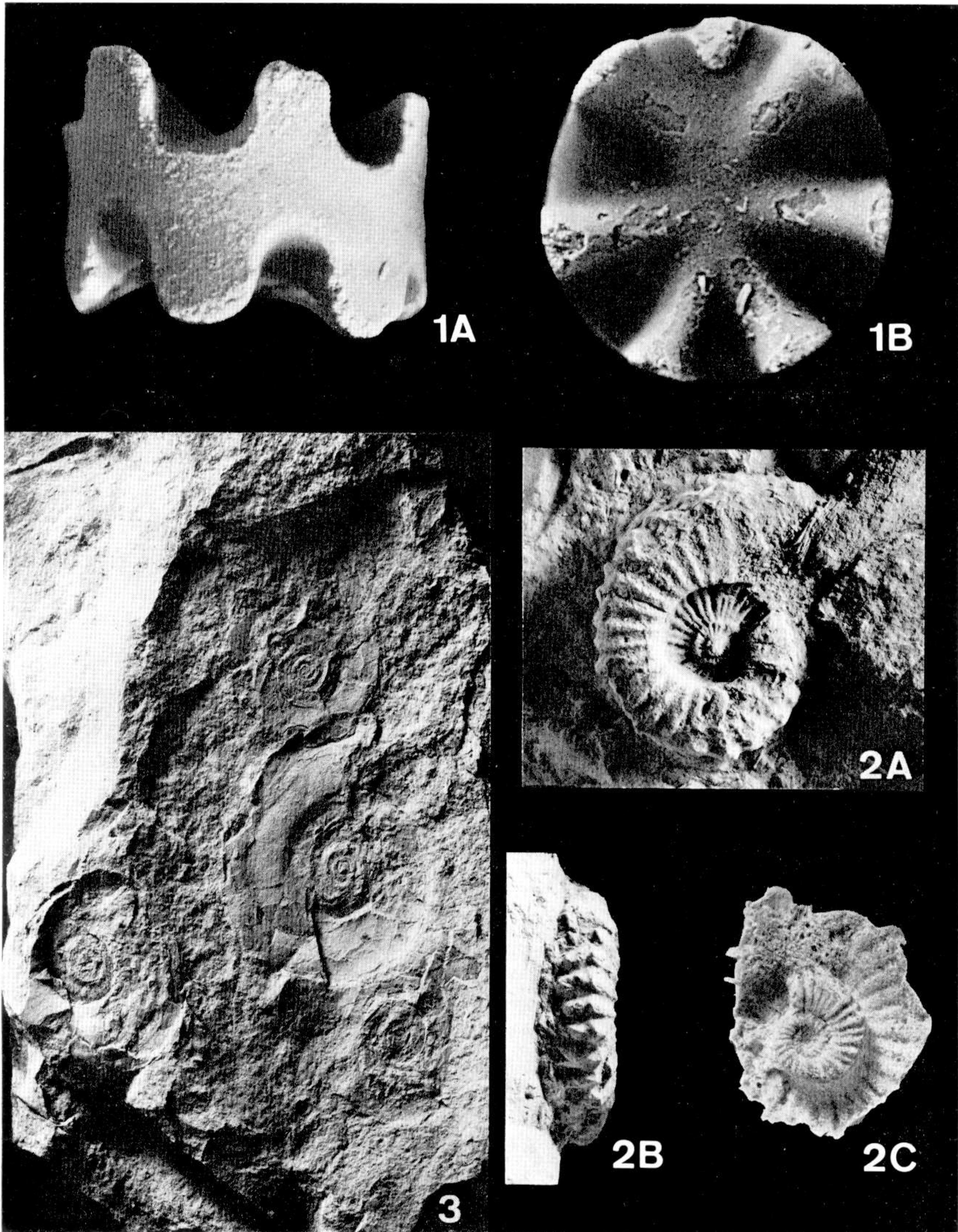
Abb. 1. Rhabdoceras suessi HAUER. Hypotypoid SMNS (Staatl. Mus. Naturkunde Stuttgart) 22760, Schicht A 22, Weißloferbach/Koessen (Tirol). A. Lateralansicht einer Kammer, B. Septalan- sicht, ca. 35/1.
