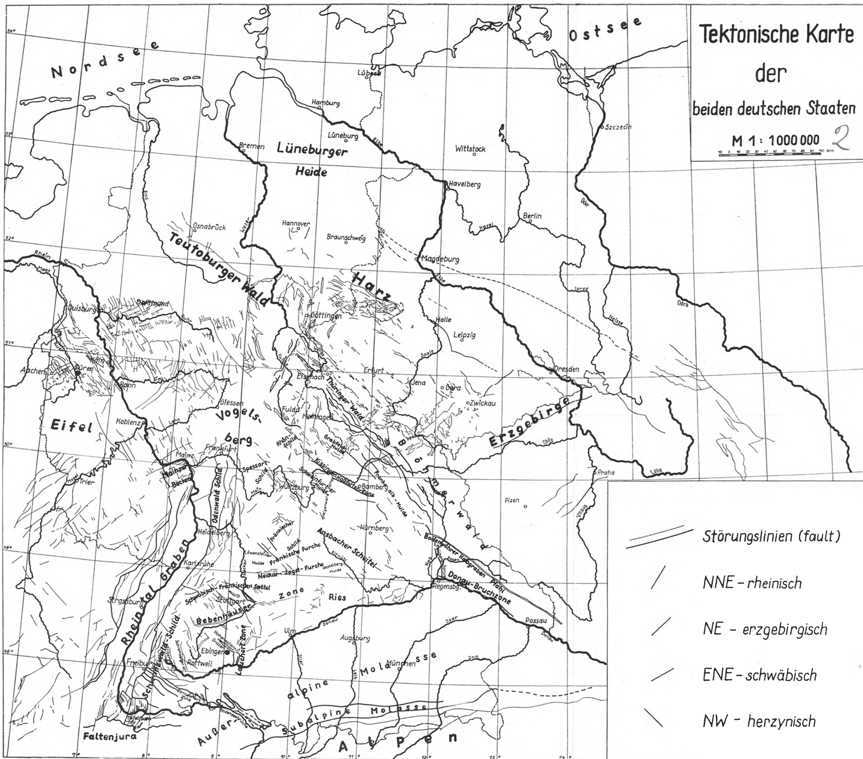
Abb. 2. Tektonische Karte der beiden deutschen Staaten
