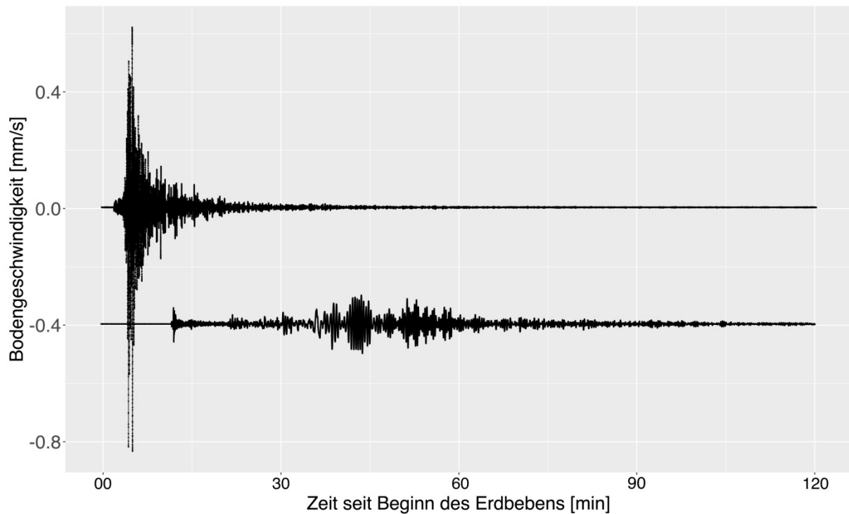
Abb. 1: Seismogramme von GTTG-Z; oben USGS-KR (Kroatien), unten USGS-AL (Alaska)
