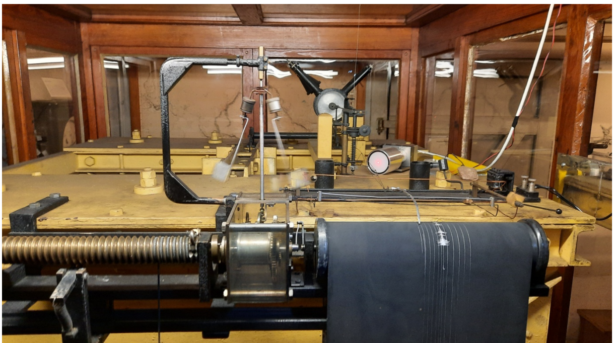
Abb. 2: Astaticher Vertikalseismograph von Wiechert, Göttinger Station GTT-Z; Foto: P. Schmitt
