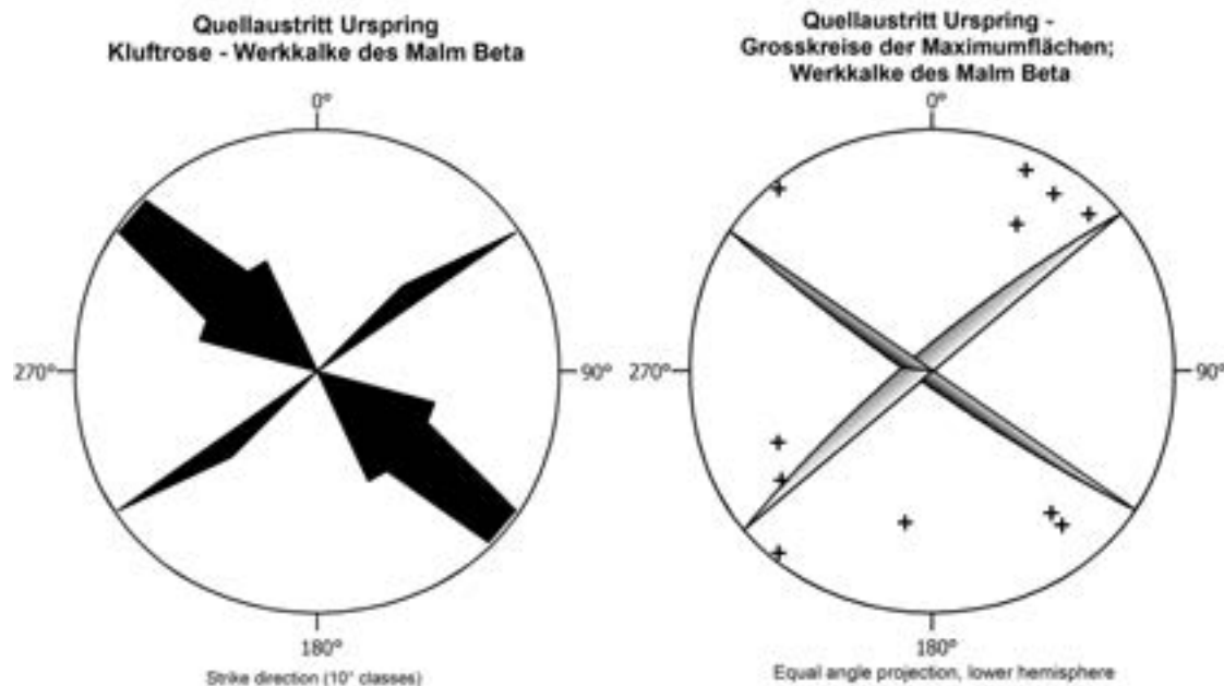
Abb. 16: Kluftröse und Großkreise der Maximumflächen in der Werkkalke (Malm Beta) des Quellmundlochs »Q_01« des »Urspring« 1650 m SSW' Hohenmirsberg/Ofr.
