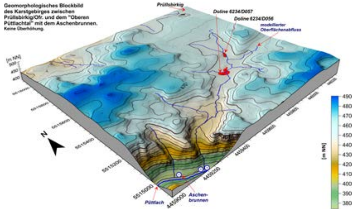
Abb. 19: 3D-Blockbild des Gebiets des Großdolinenfeldes SSW' Prüllsbirkig/Ofr. mit den Trockentälern, den Großdolinen und den modellierten Abflussrinnen bis zum »Oberem Püttlachtal« mit dem »Aschenbrunnen«.
