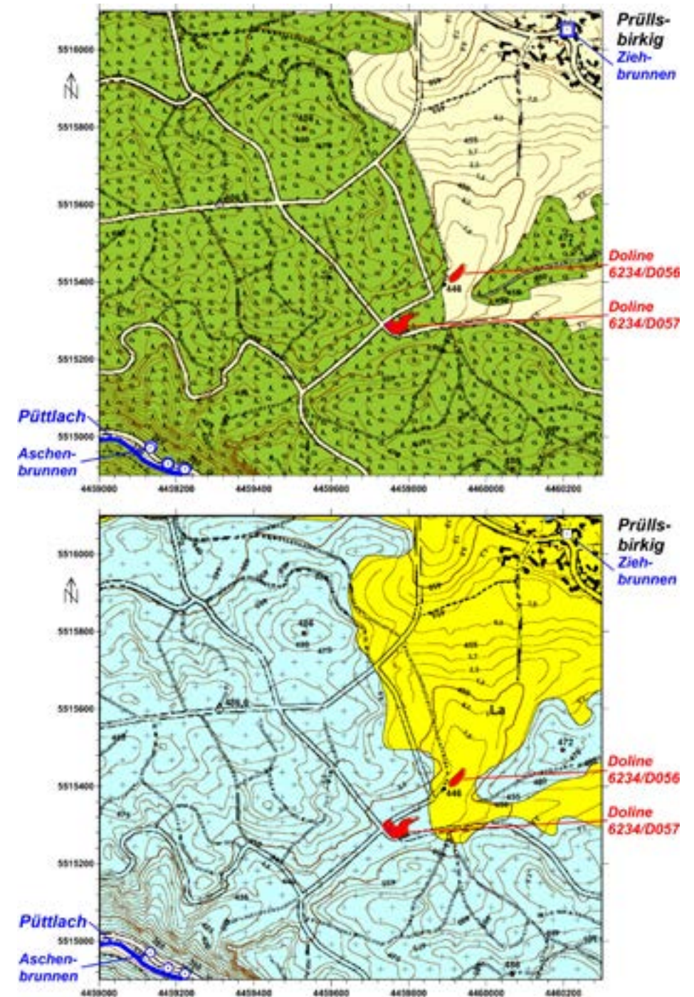
Abb. 17: Topographische (oben) und geologische (unten) Spezialkarte des Großdolinenfeldes SSW' Prüllsbirkig/Ofr. bis hin zum »Oberen Püttlachtal« mit dem »Aschenbrunnen«; Erläuterung siehe Text.
