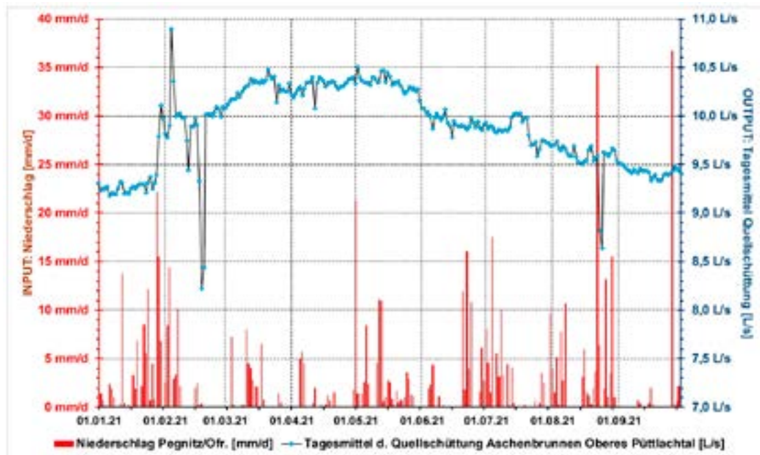
Abb. 20: Tagessummen der während der 9-monatigen Periode vom 01.01.2021 bis 01.10.2021 in der Wetterstation Pegnitz/Ofr. registrierten Niederschläge [mm/d] sowie Tagesmittel der beobachteten Quellschüttungsraten des Aschenbrunnen im Oberen Püttlachtal E' Pottenstein/Ofr.; Rohdatengrundlage: LFU (2021).
