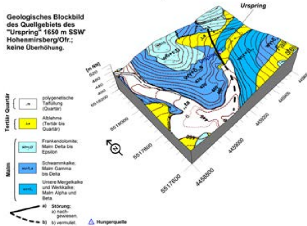
Abb. 13: Geomorphologisches (oben) und geologisches (unten) 3D-Blockbild des Haupt- und Nebentrockentales im Quellgebiet des »Urspring« 1650 m SSW Hohenmirsberg/Ofr.; Erläuterung siehe Text.
