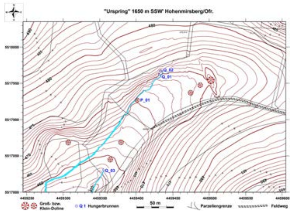
Abb. 14: 3D-Blockbild (oben) und Vermessungskarte des unmittelbaren Quellenbereichs des »Urspring« 1650 m SSW Hohenmirsberg/Ofr. nebst den Hungerquellen Q_01 bis Q_03, dem Ponor P_01, den temporären Wasserläufen und den diversen Groß- und Kleindolinen.
