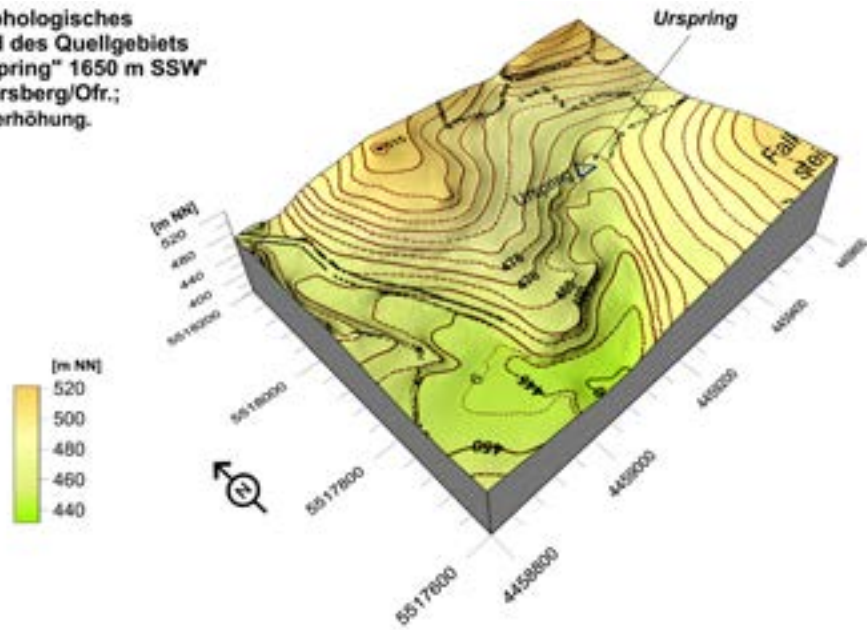
Geologisches Blockbild des Quellgebiets des "Urspring" 1650 m SSW Hohenmirsberg/Ofr.; keine Überhöhung.
